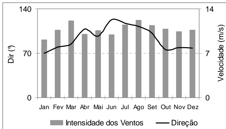
Figura 3. Variação mensal das características de ventos (velocidade e direção) na região do estuário de Diogo Lopes (INMET, 2010).
