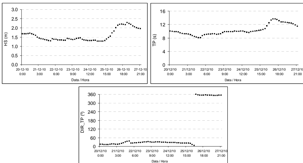
Figura 10 - Valores de HS, TP e DIR_TP do modelo de 3ª geração WWIII, 20 de 27 de Dezembro de 2010, para o ponto da malha 3°S36°W.
