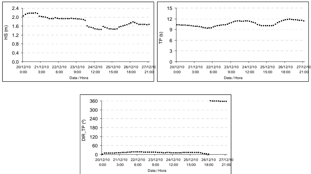
Figura 11 - Valores de HS, TP e DIR_TP do modelo de 3ª geração WWIII, 15 a 22 de Fevereiro de 2011, para o ponto da malha 3°S36°W
