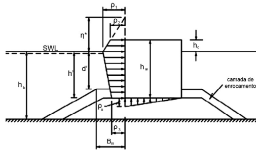
Figura 17 – Método de Goda (Fonte: Coastal Engineering Manual, 2006).
