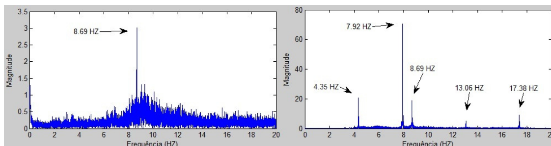
Figura 4- Análise do processo de atracação usando a FFT.
