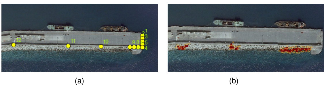
Figura 3 – (a) Distribuição espacial dos pontos de controlo pertencentes à rede de monitorização da Estabilidade Absoluta do Quebramar; (b) Subconjuntos de Tetrápodes (Pereira et al., 2011).
