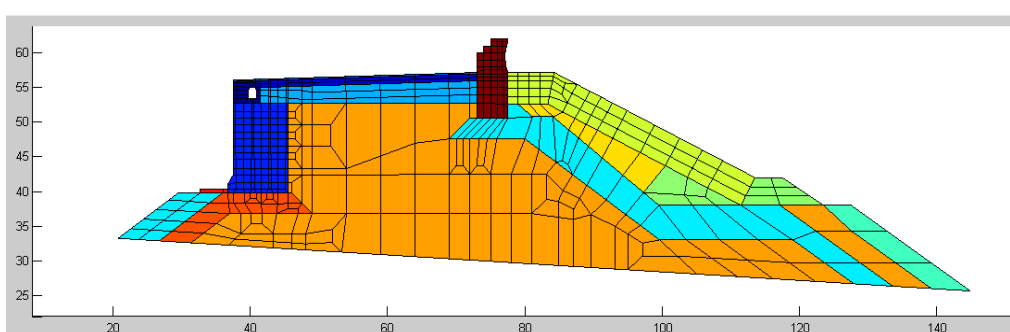
Figura 15 – Perfil do quebramar. Representação das camadas com diferentes materiais.
